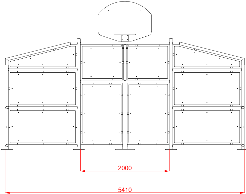
ALZADO
